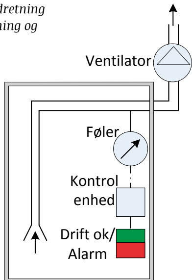
Kontrolanordning med føler og alarmsignal ved 1 punktudsug
