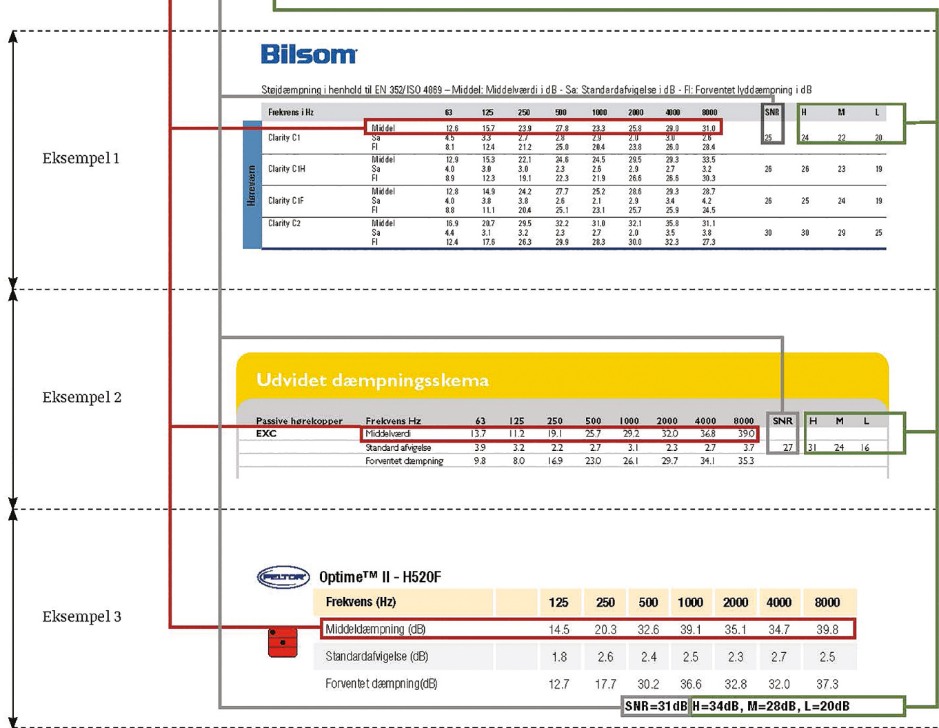
Figuren viser uddrag fra datablade for 3 forskellige høreværn. Hvert datablad indeholder de krævede 3 forskellige oplysninger om dæmpningen. Hver type af oplysning er indrammet med henholdsvis rød, grøn og grå farve.
